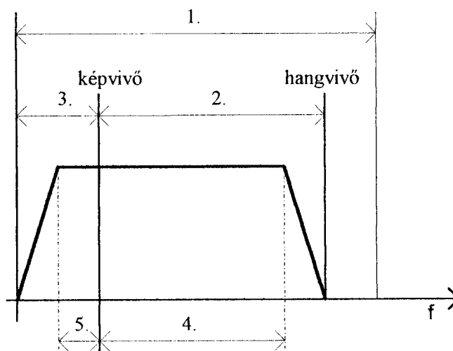
A kisugárzott tv-jel egyes jellemzőinek értelmezése (a táblázat sorszámaival jelölve)
