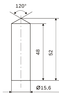
2. ábra: Hengeres bronzdugattyú, méreték mm-ben
