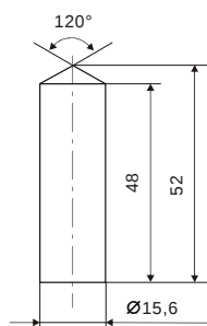
2. ábra: Hengeres bronzdugattyú, méretetek mm-ben
