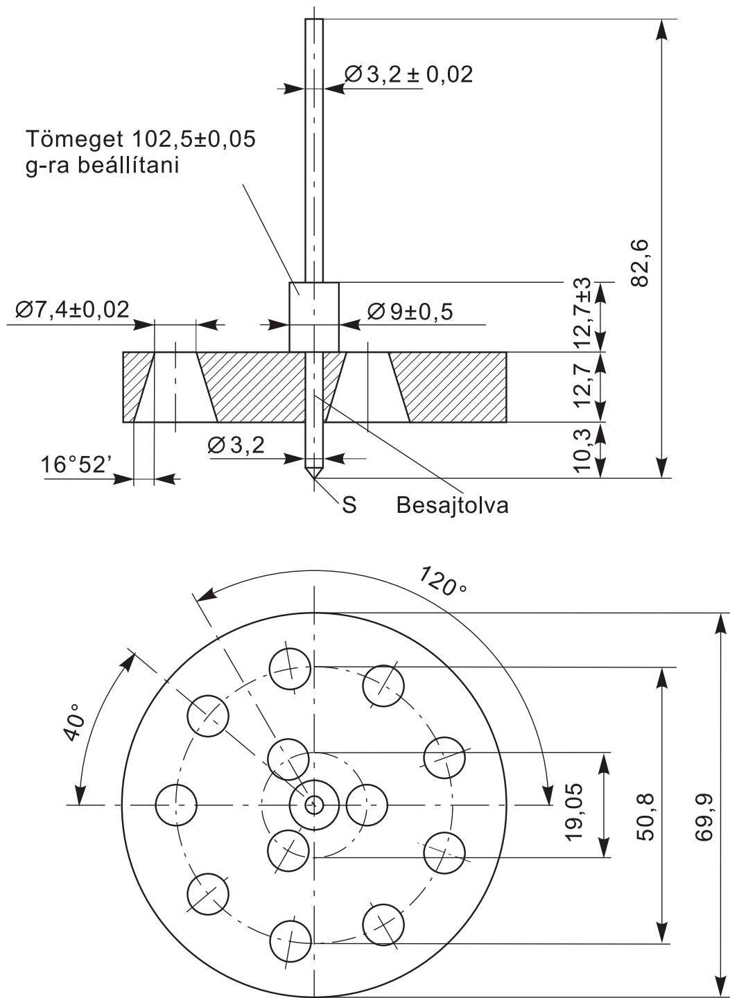
4. ábra: Penetrométer
