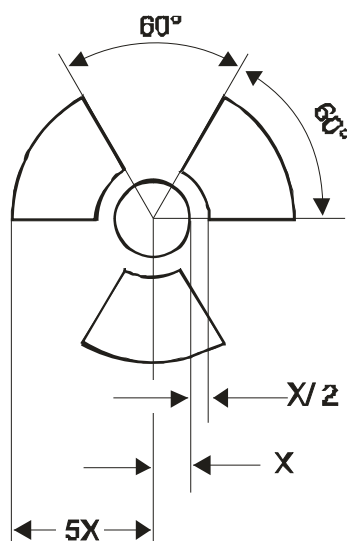
Sugárveszély szimbólum
