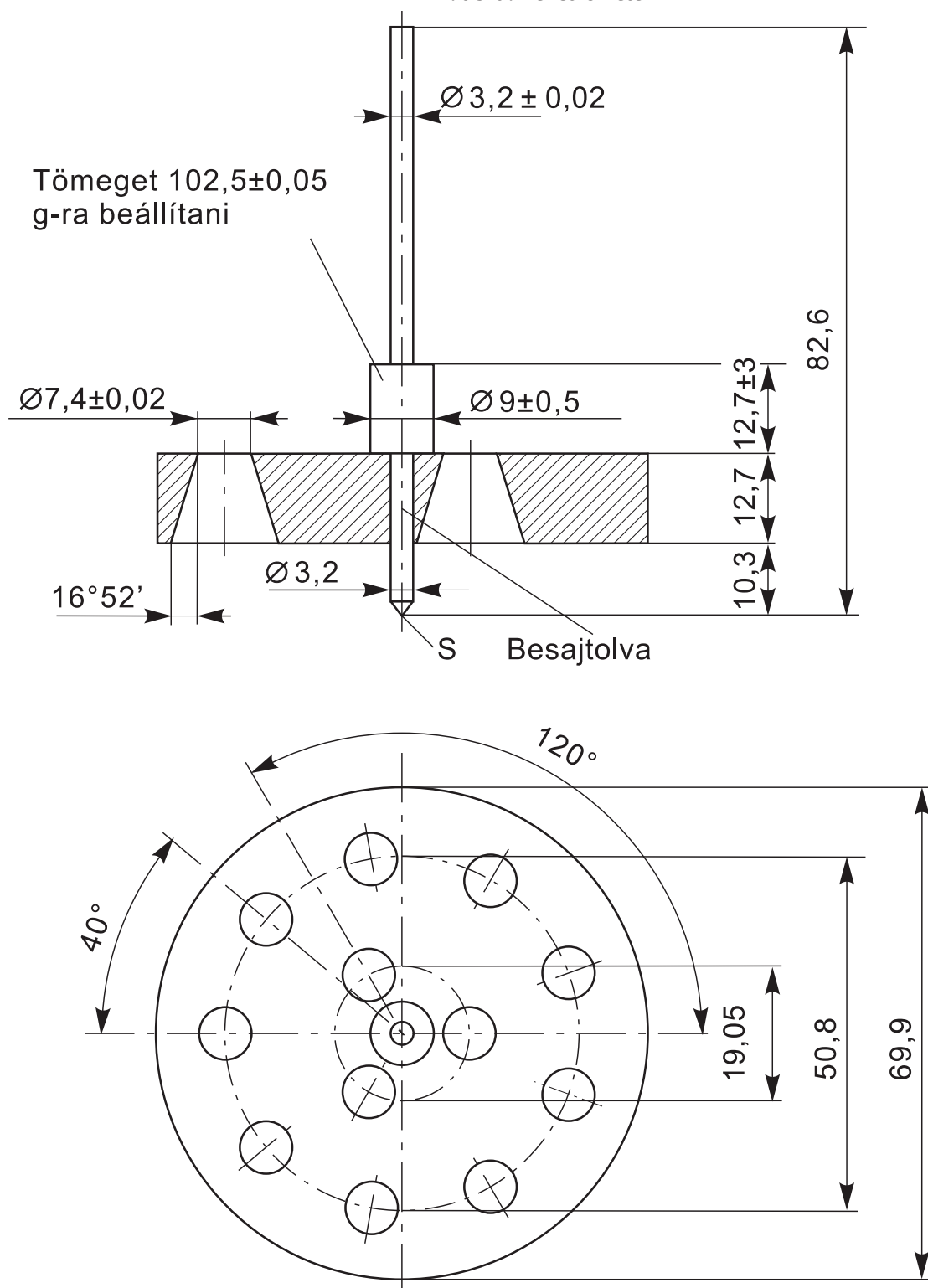
4. ábra: Penetrométer
