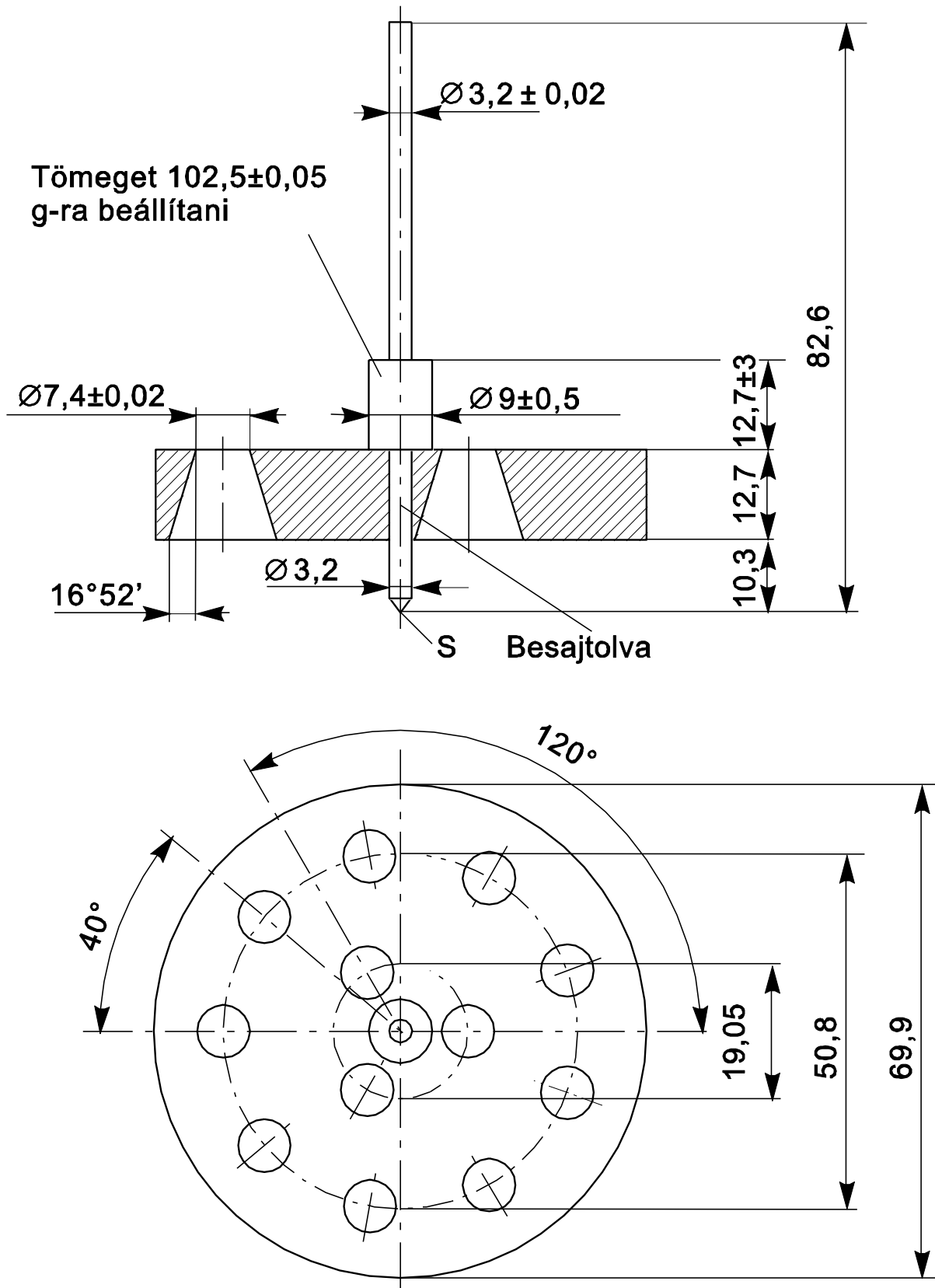
4. ábra: Penetrométer
