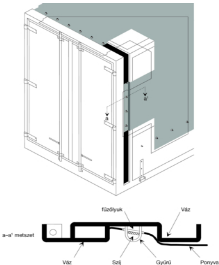
7. számú vázlat Speciálisan kialakított vázhoz rögzített ponyva mintája
