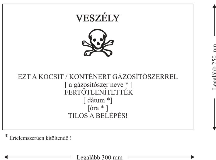
Gázosítószeres fertőtlenítésre figyelmeztető jelölés
