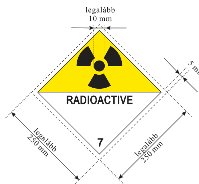
7D sz. nagybarca a 7 osztály radioaktív anyagaihoz
