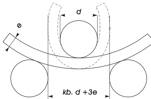
A hajlítási próba vázlata
