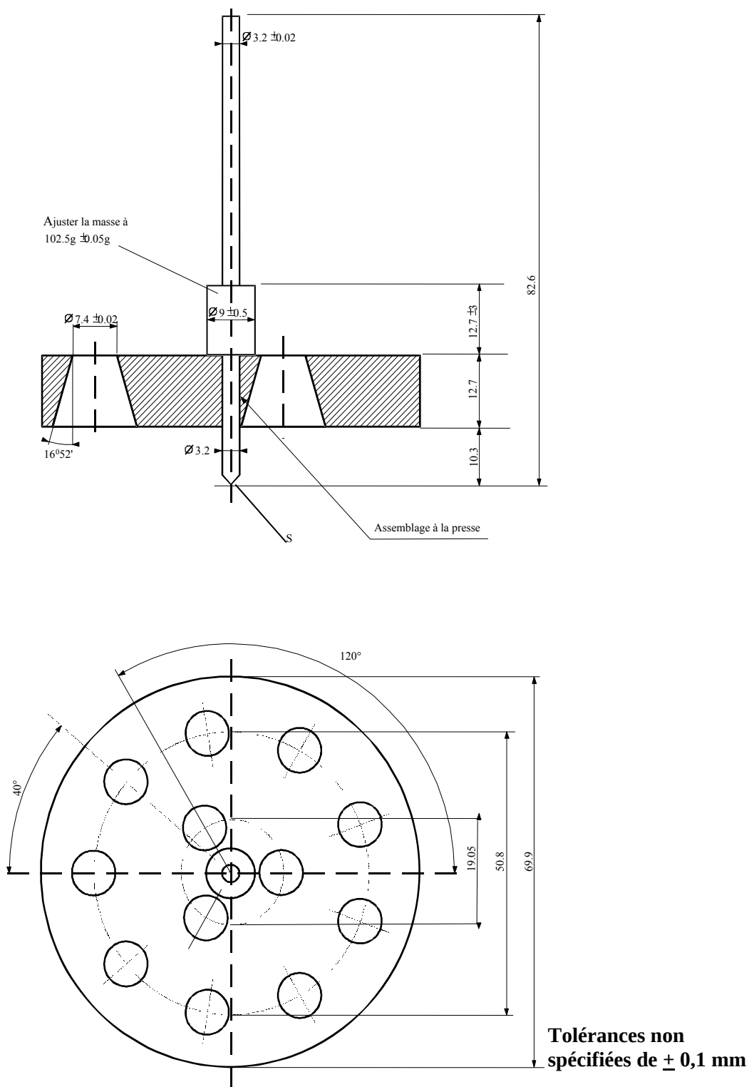
Figure 1 – Pénétromètre
