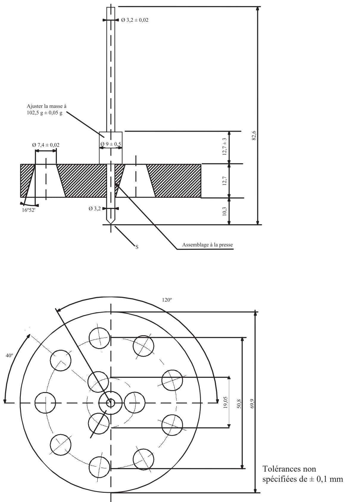
Figure 1 – Pénétromètre
