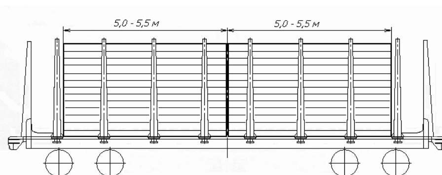
77. ábra / 5,0 – 5,5 m hosszú faanyagok elhelyezése
