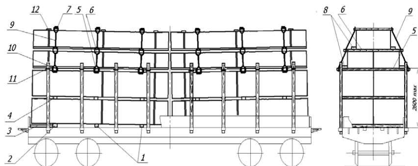
52. ábra – Fűrészárúkötegek pórekocsin történő elhelyezése
