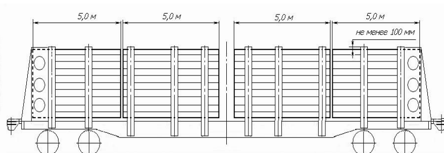
87. ábra – az 5,0 m-t meghaladó hosszúságú faáru elhelyezésének módja
