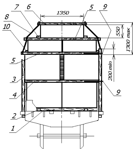
Рисунок 59 – Размещение пакетов на платформе по варианту 3
