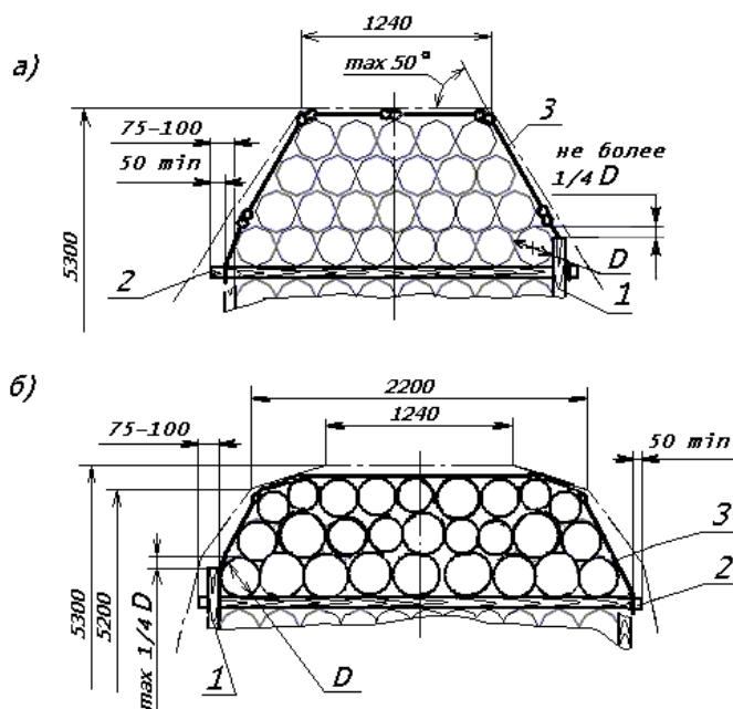
Рисунок 9 – «Шапка», сформированная:
