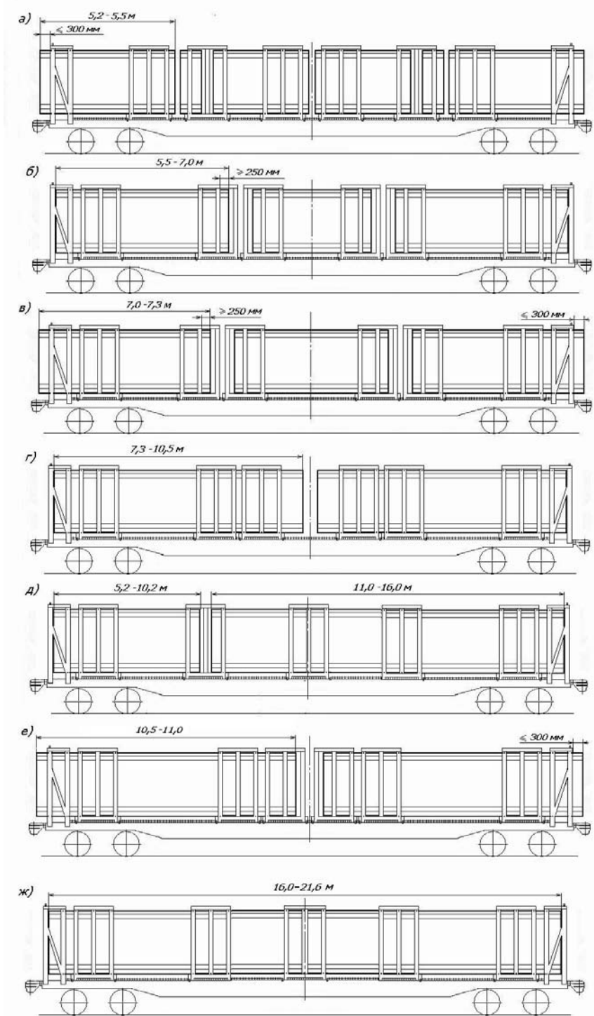
99. ábra / 5,2 m és ennél hosszabb faanyagok elhelyezése
