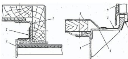
7.5-14 sz. ábra Az ajtónyílás-küszöb tömítése:
