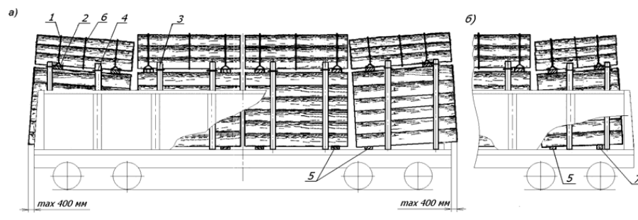
3. ábra – Gömbfák elhelyezése és rögzítése négy rakásban az alapprakszelvényen belül:
