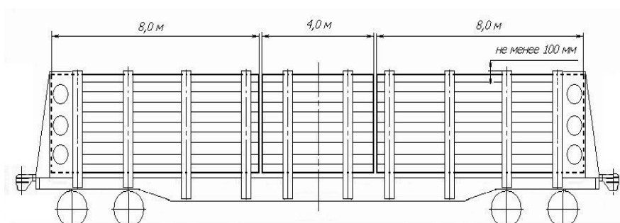
91. ábra – a 4,0 m és 8,0 m-es hosszúságú faáru együttes elhelyezésének módja
