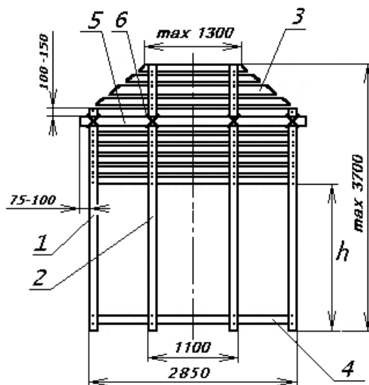
14. ábra – Homlokpajzs
