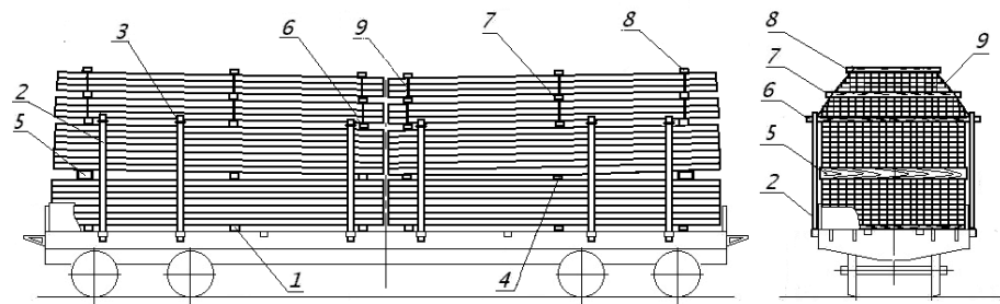
34. ábra – Kötegetlen fűrészáru pórekocsin 1 – alátét; 2 – támasz; 3 – feszítőelem; 4 – közbetét; 5 – vastagított közbetét; 6 – hosszabbított közbetét; 7 – „süveg” közbetétje; 8 – felső keresztléc; 9 – „süveg” kötőőleme
