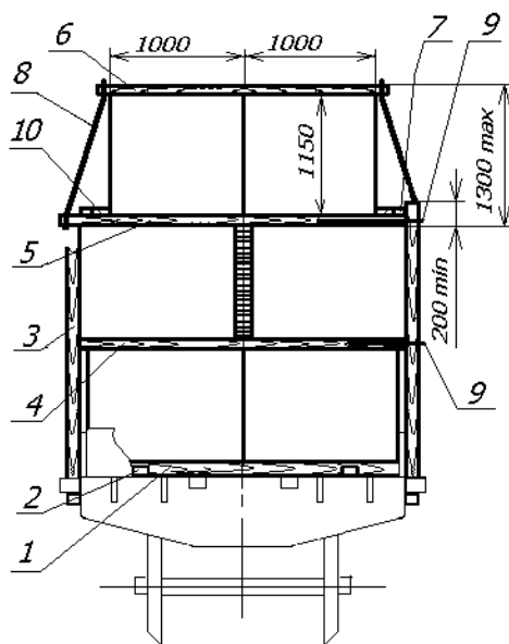
Рисунок 55 – Размещение пакетов на платформе по варианту 1
