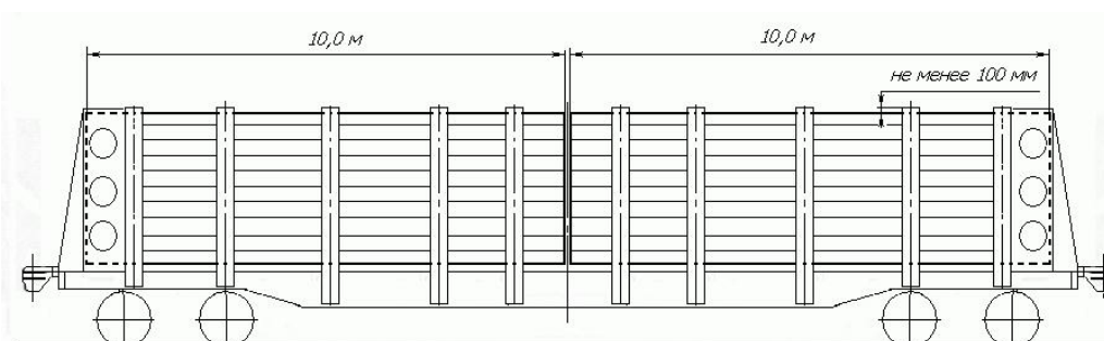
Рисунок 89 – Размещение лесоматериалов длиной 10,0 м
