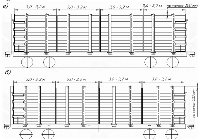
71. ábra / 3,0 – 3,2 m hosszú faanyag elhelyezése
