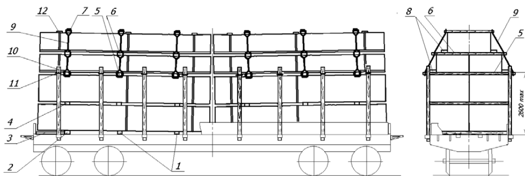
Рисунок 52 – Размещение пакетов пиломатериалов на платформе
