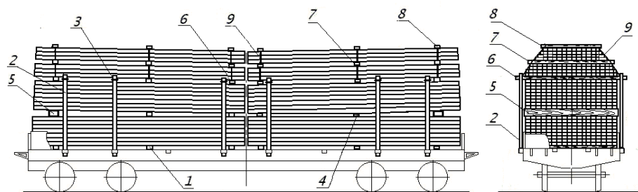
Рисунок 34 – Непакетированные пиломатериалы на платформе
