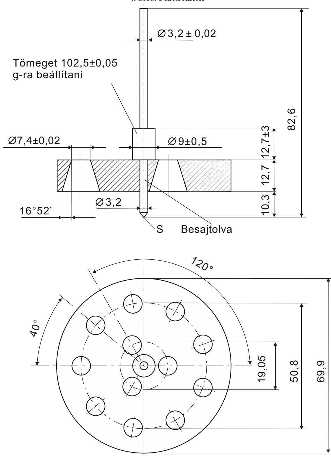
4. ábra: Penetrométer
