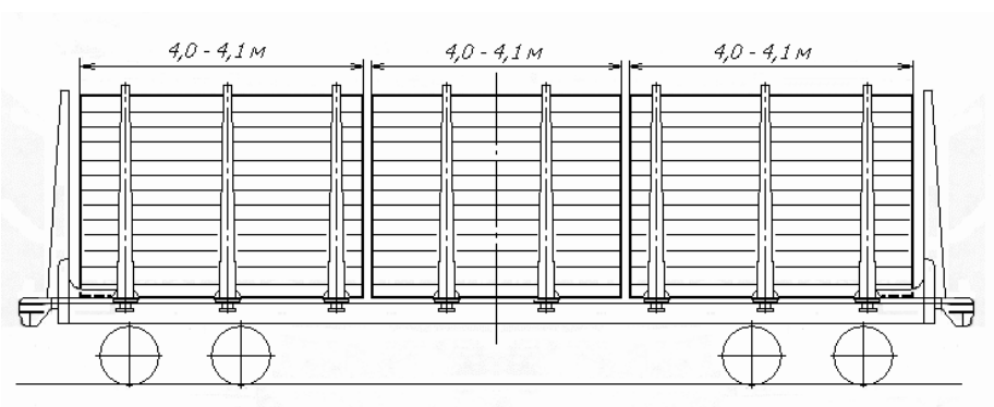
76. ábra / 4,0 – 4,1 m hosszú faanyagok elhelyezése
