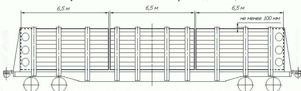
Рисунок 88 – Размещение лесоматериалов длиной 6,5 м
