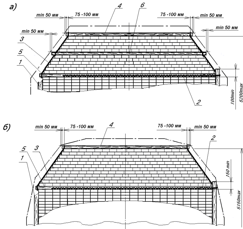
Рисунок 37 – Максимальные допускаемые размеры «шапки»:
