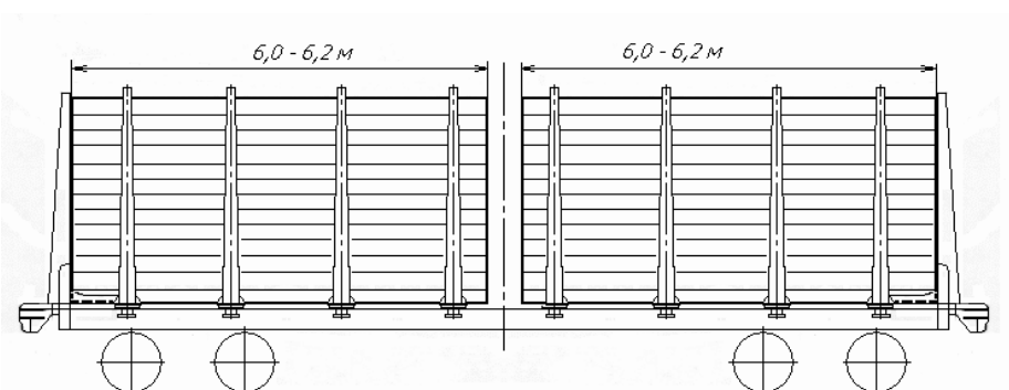
78. ábra / 5,0 – 6,2 m hosszú faanyagok elhelyezése
