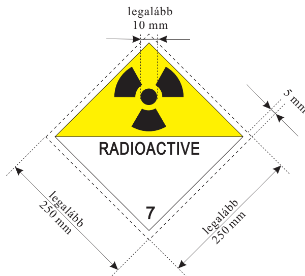
7D sz. nagybárca a 7 osztály radioaktív anyagaihoz
