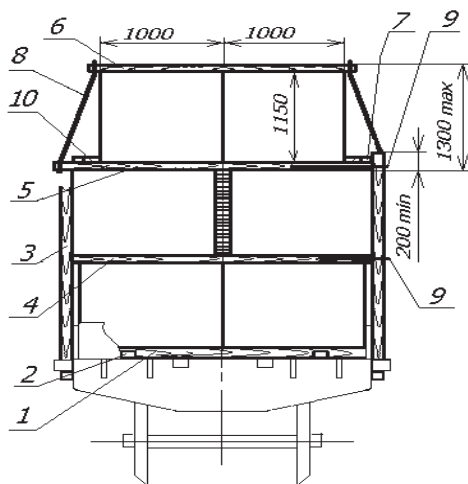
55. ábra – Kötegek 1-es változat szerinti elhelyezése pórekocsin
