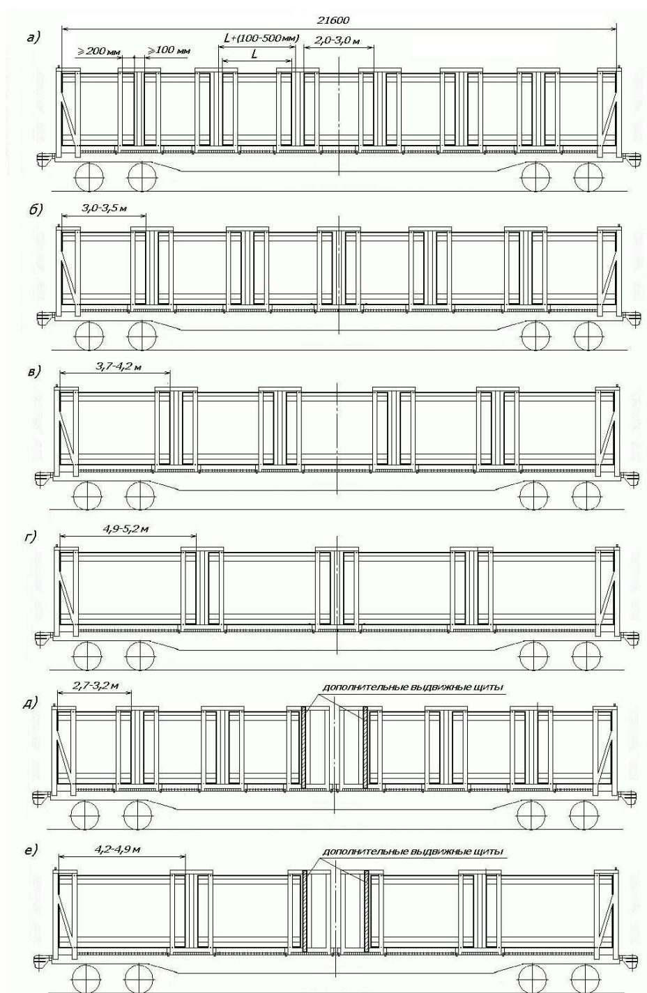
Рисунок 98 – Размещение лесоматериалов длиной 2,0 – 5,2 м (L – длина штабеля)
