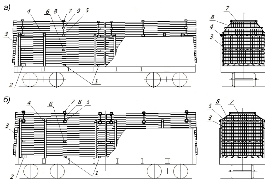
Рисунок 35 – Непакетированные пиломатериалы в полувагоне:
