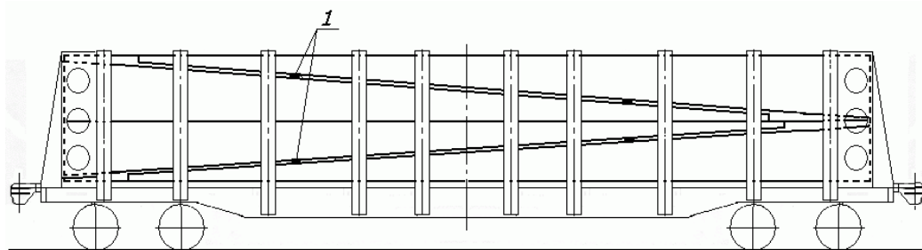
Рисунок 92 1 – прокладка
