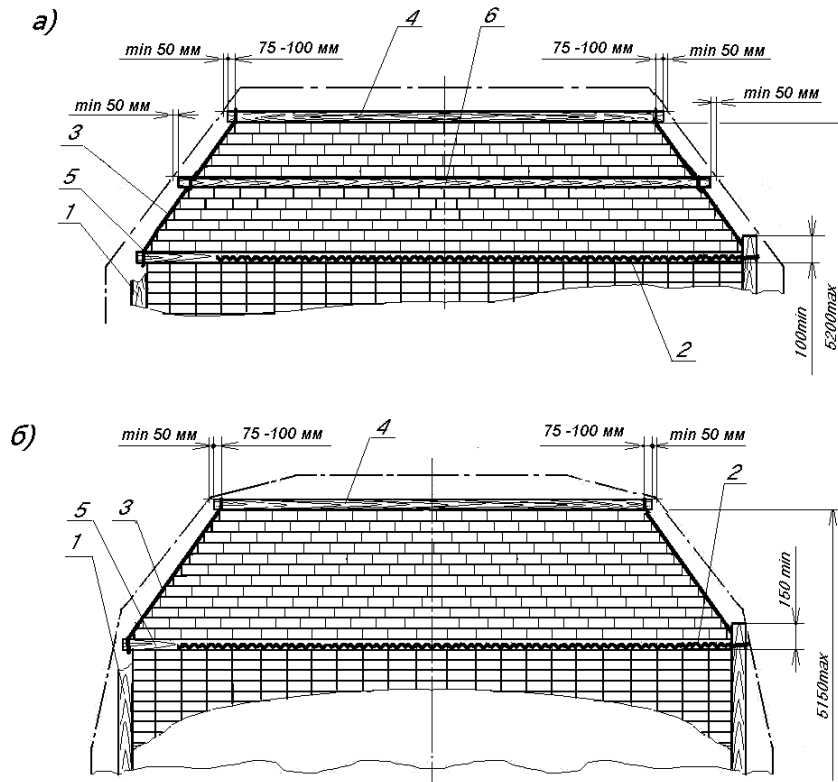
37. ábra – A „süveg” megengedett legnagyobb méretei:
