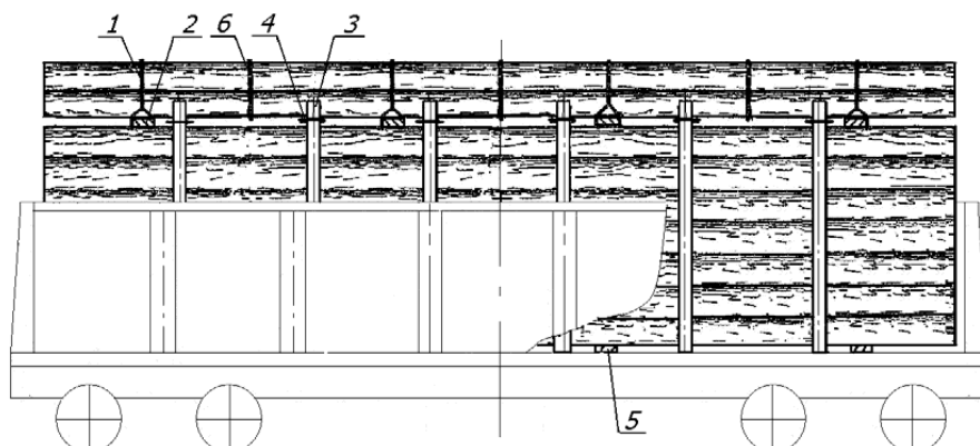
Рисунок 8 – Размещение и крепление круглых лесоматериалов одним штабелем
