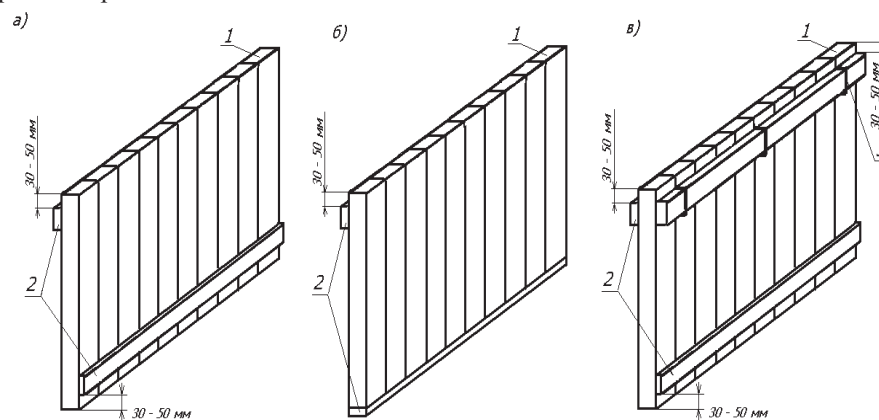
43. ábra – Homlokpajzs:
