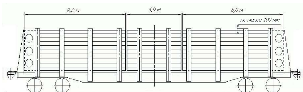
Рисунок 91– Размещение лесоматериалов длиной 4,0 м и 8,0 м совместно
