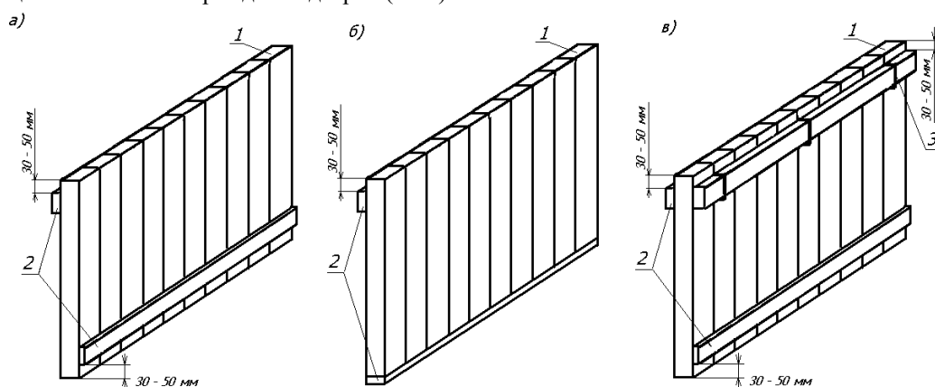
Рисунок 43 – Торцевой щит: а), б) для крепления пакетов непропитанных шпал; в) для крепления пакетов пропитанных шпал 1 – шпала; 2 – доска; 3 – увязка
