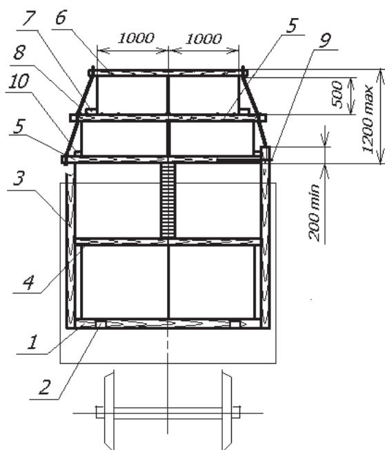
56. ábra – Kötégek 2-es változat szerinti elhelyezése nyitott kocsin 1 – vastagított alátét; 2 – támaszték; 3 – támasz; 4 – közbetét; 5 – hosszabbított közbetét; 6 – leszorító lécz; 7, 10 – távtartó deszka; 8 – lekötő szerkezet; 9 – feszítőelem;
