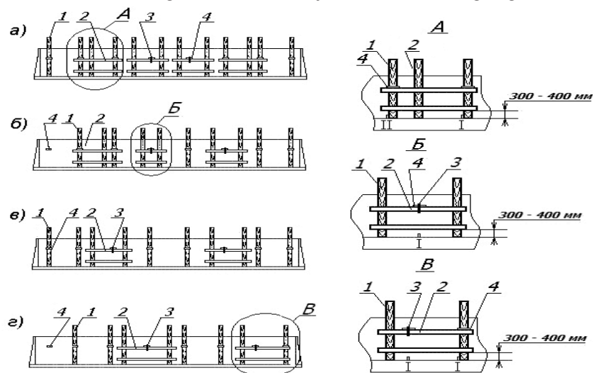
1. ábra – Példák támaszok nyitott kocsin történő elhelyezésére kötegetlen faanyagok szállítása esetén:
