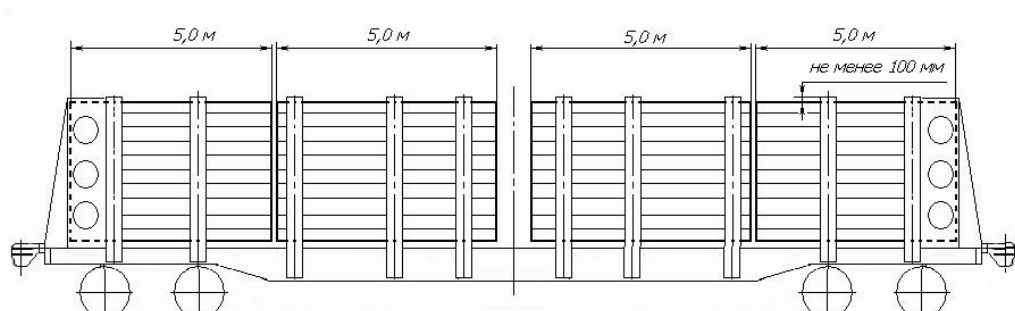
Рисунок 87 – Размещение лесоматериалов длиной 5,0 м
