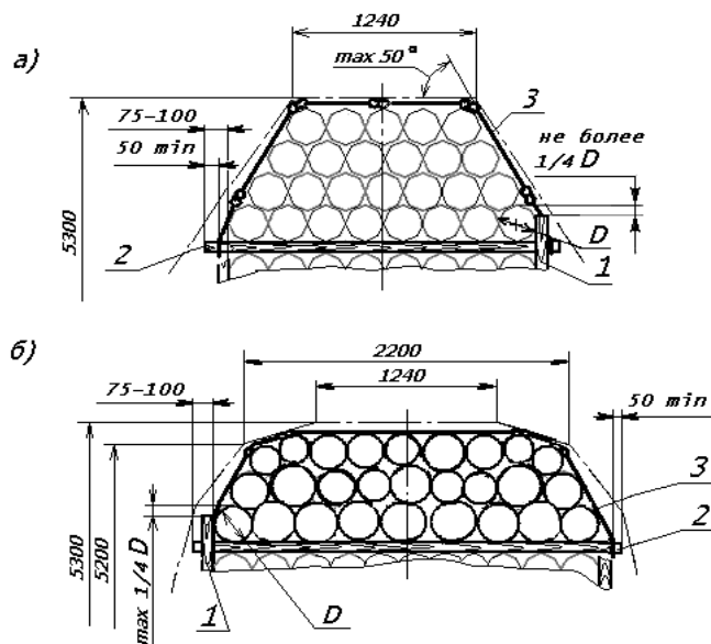
9. ábra – Kialakított „süveg”:
