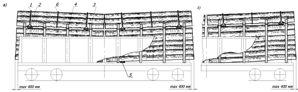
7. ábra – Gömbfák elhelyezése és rögzítése két rakásban, nyitott ajtajú nyitott kocsin:
