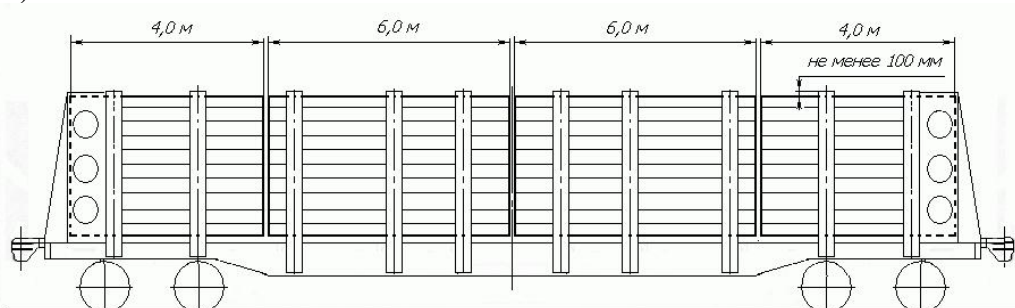
Рисунок 90 – Размещение лесоматериалов длиной 4,0 м и 6,0 м совместно
