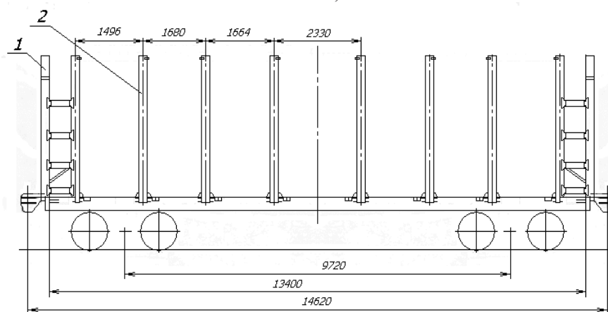
80. ábra 1-homlokzati fal, 2 – oldalkeret
