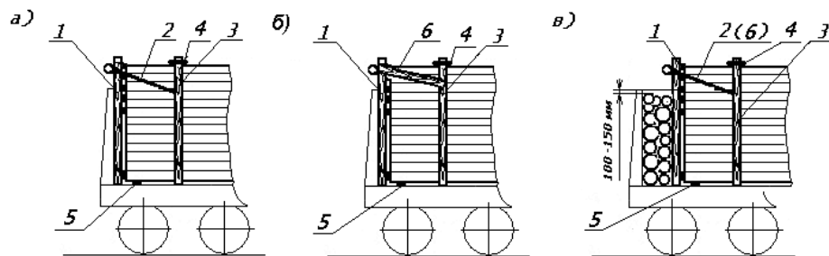
12. ábra – Homlokpajzsok elhelyezése a nyitott kocsin:
