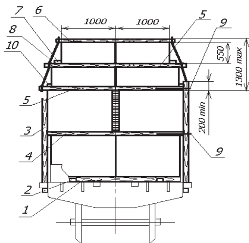
56. ábra – Kötégek 2-es változat szerinti elhelyezése nyitott kocsin 1 – vastagított alátét; 2 – támaszték; 3 – támasz; 4 – közbetét; 5 – hosszabbított közbetét; 6 – leszorító lécz; 7, 10 – távtartó deszka; 8 – lekötő szerkezet; 9 – feszítőelem;
