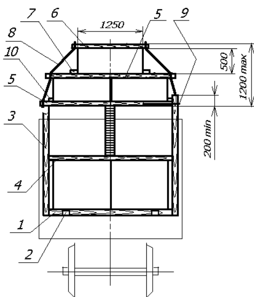
Рисунок 58 – Размещение пакетов в полувагоне по варианту 3
