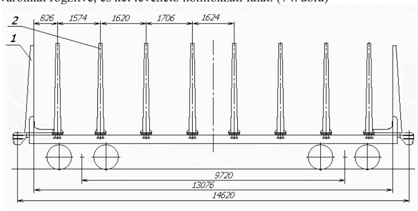
74. ábra 1 - homlokfál, 2 - oldalkeret
