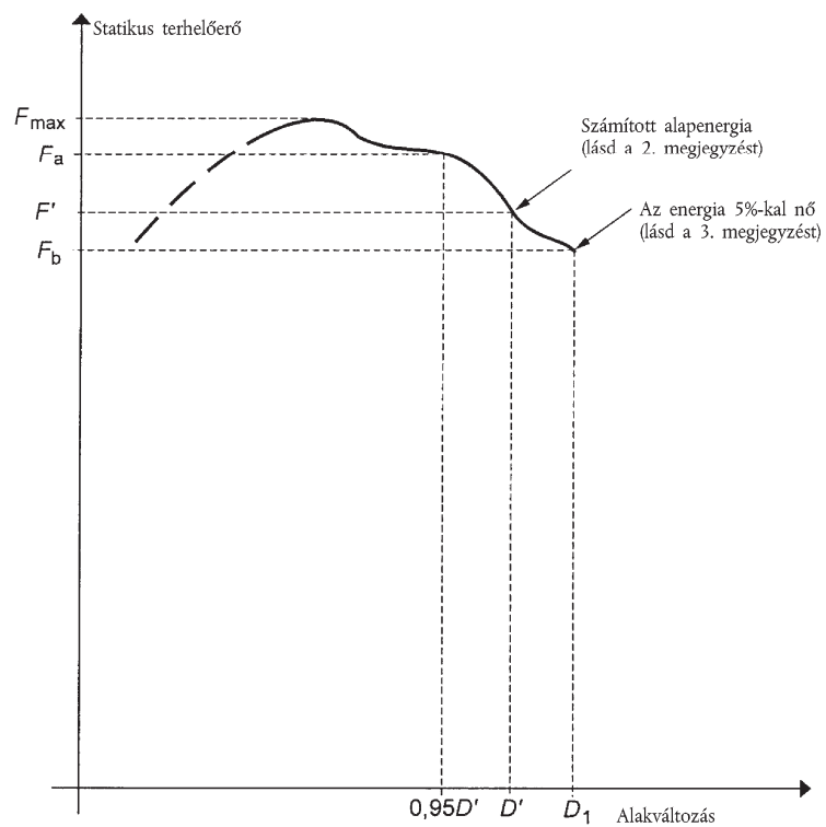
6.19. ábra Erő-alakváltozás görbe Túlterhelési vizsgálat szükséges
