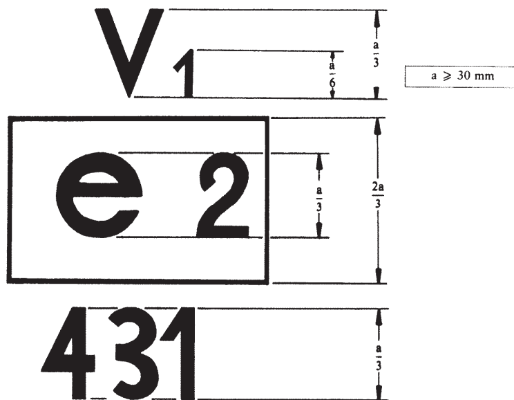
Példa az EU-alkatrész-típus-jóváhagyási jelre
