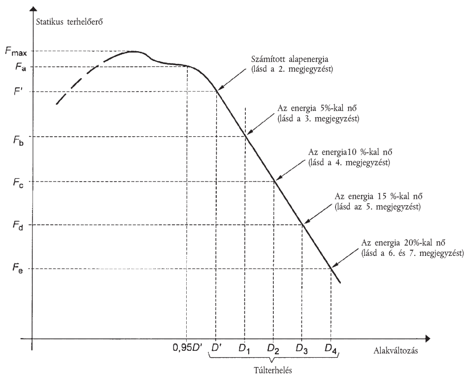
6.20. ábra Erő-alakváltozás görbe A túlterhelési vizsgálatot folytatni kell
