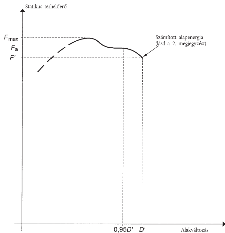
6.18. ábra Erő-alakváltozás görbe Túlterhelési vizsgálat nem szükséges
