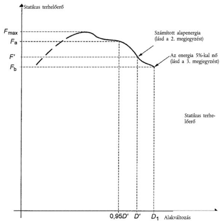
7.10. ábra Erő-alakváltozás görbe Túlterhelési vizsgálat szükséges
