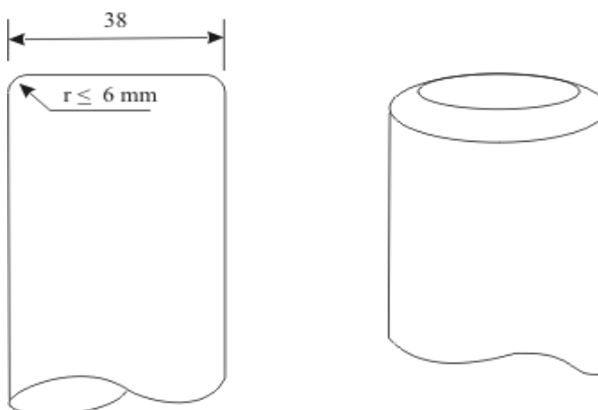
méretetek mm-ben 6.3.5.4.2 ábra
